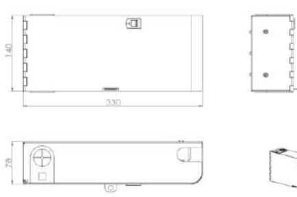
Caja de empalme con capacidad 2 placas
