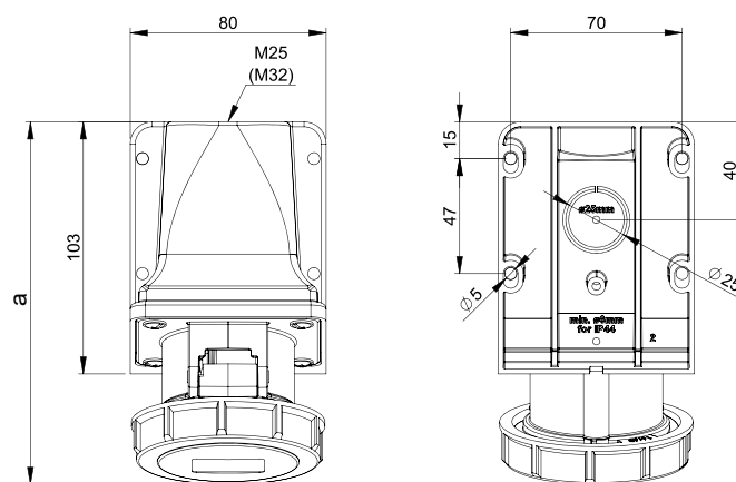
IP67 - 16A-32A
