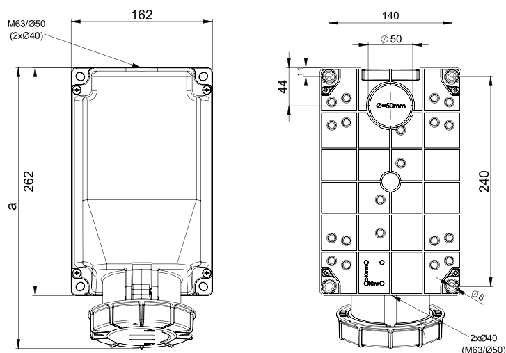
IP67 - 125A
